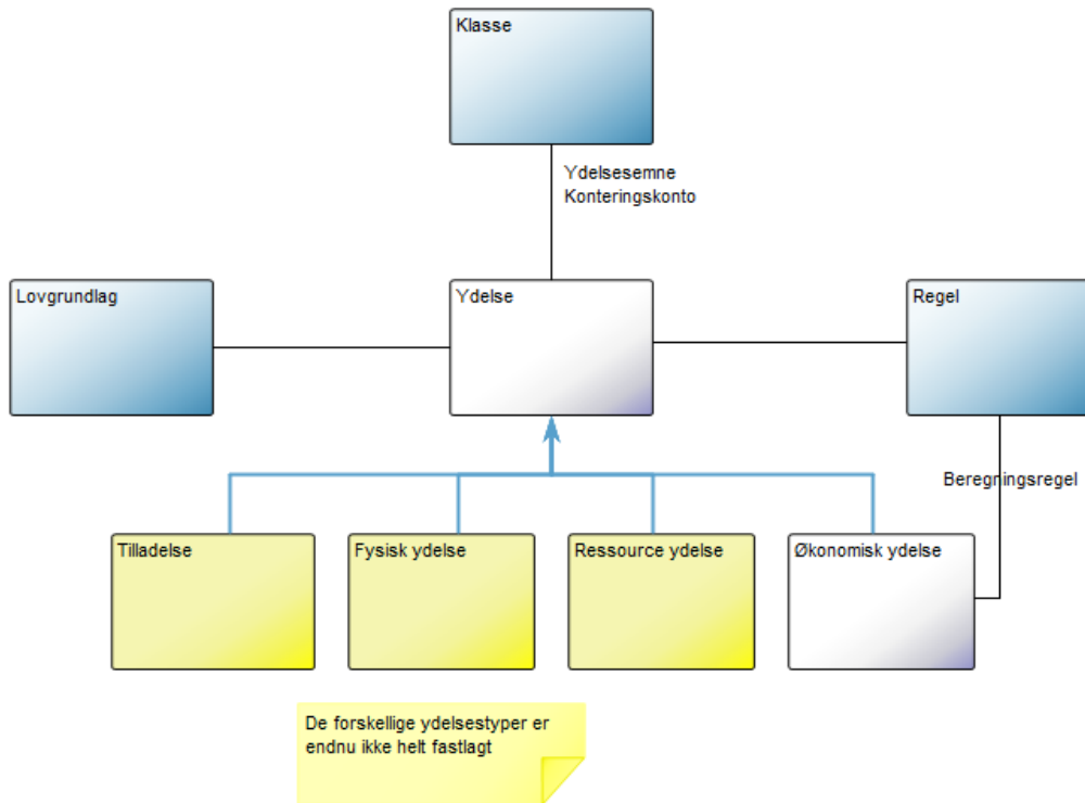
Figur 1 - Objektmodel for byggeblok Ydelse
